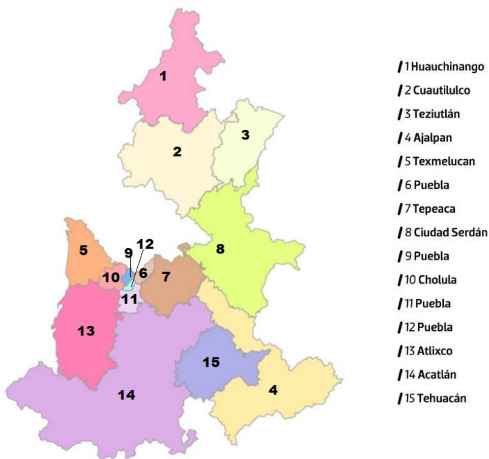
Figura 2. Distritos electorales del Estado de Puebla. Fuente: Instituto Nacional Electoral (INE) (2017).
